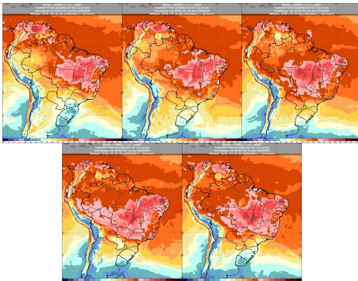
Figura 2: Previsão de temperatura máxima de 11 a 15 de maio de 2026 às 15h (horário de Brasília). Fonte: INMET
