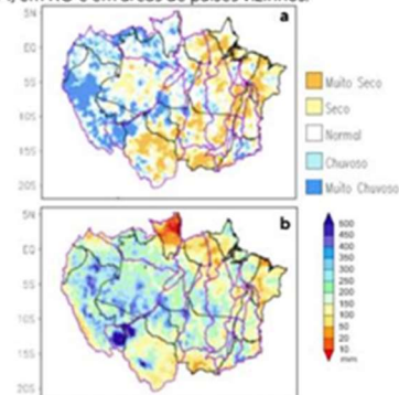
Figura 1. Anomalia Categorizada (a) e chuva acumulada (b) para janeiro de 2026. Dados do MERRA/CPTEC processados pelo Censipam.
