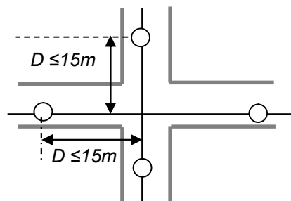
Figura 2 – Cruzamento Aéreo
